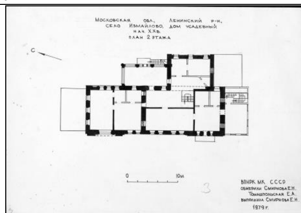
Усадьба "Троицкое". Главный дом. План 2-ого этажа
