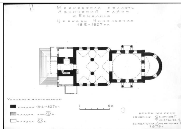
Церковь Никольская. План
