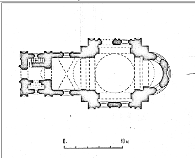
Церковь Ильи пророка. План
