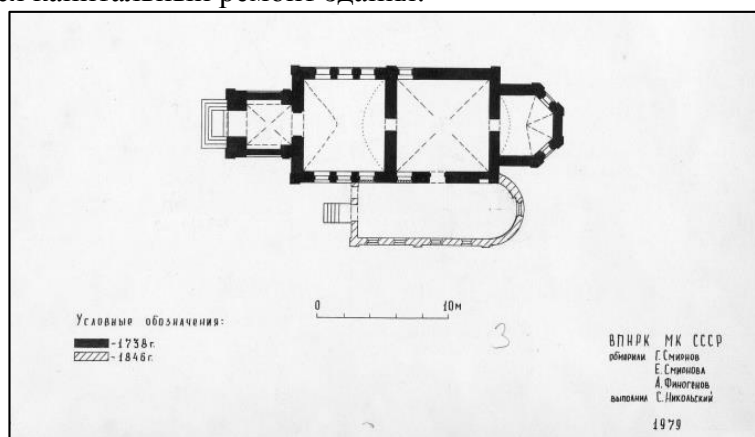
План церкви
